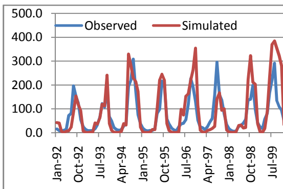
Hình 6. Dòng chảy bình quân tháng mô phỏng và thực đo tại trạm sông Lũy (1992 -1999).
