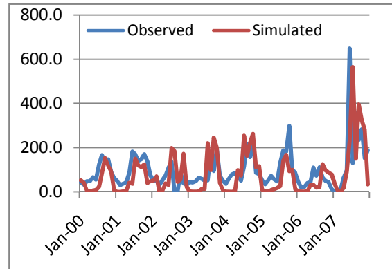
Hình 7. Dòng chảy bình quân tháng mô phỏng và thực đo tại Bình Thuận (2000 -2007).
