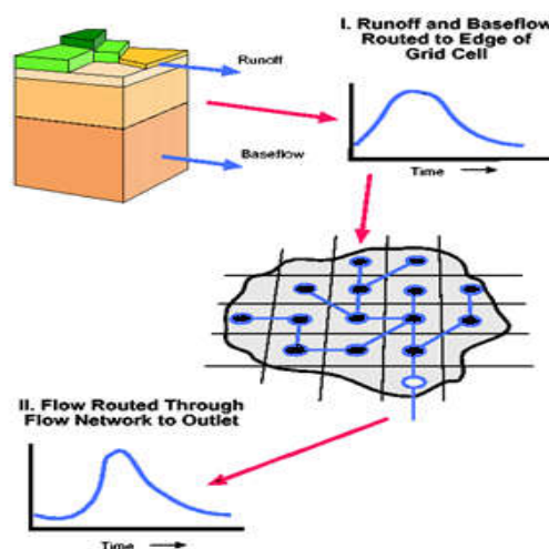
Hình 2. Sơ đồ mô phỏng tính toán dòng chảy.
