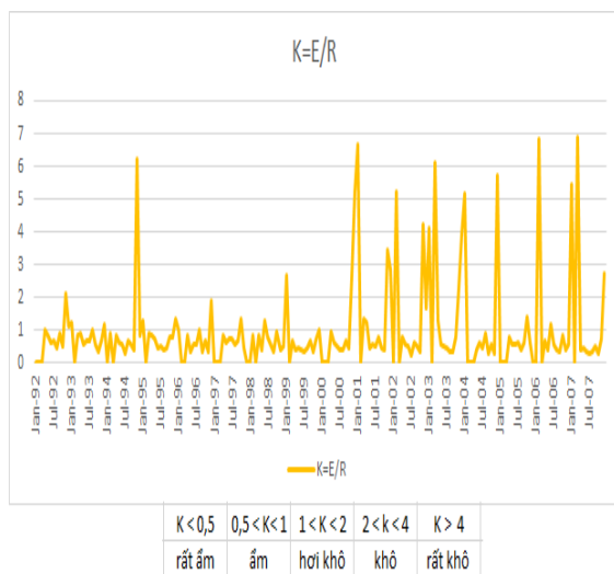
Hình 9. Diễn biến hạn theo chỉ số K (1992 – 2007).
