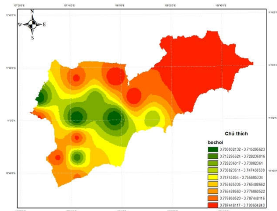
Hình 11. Phân bố lượng bốc hơi tiềm năng trung bình nhiều năm.
