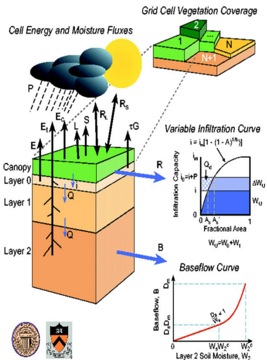
Hình 1. Cấu trúc hoạt động mô hình thủy văn VIC.
