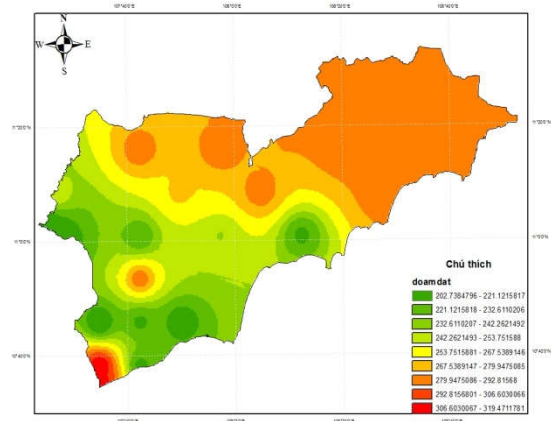
Hình 10. Phân bố độ ẩm đất trung bình nhiều năm.
