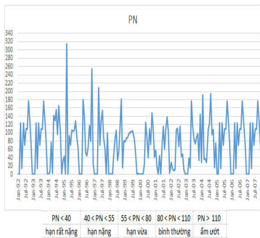
Hình 8. Diễn biến hạn theo chỉ số PN (1992 - 2007).
