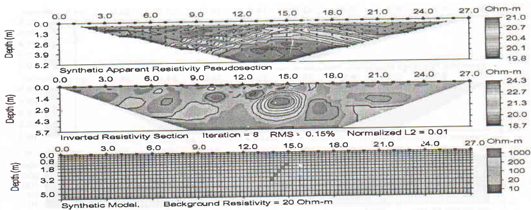
Hình 5. Tính lý thuyết khe nứt nghiêng 45^\circ , h = 1,4\text{m} đối với hệ cực dipole-dipole.
