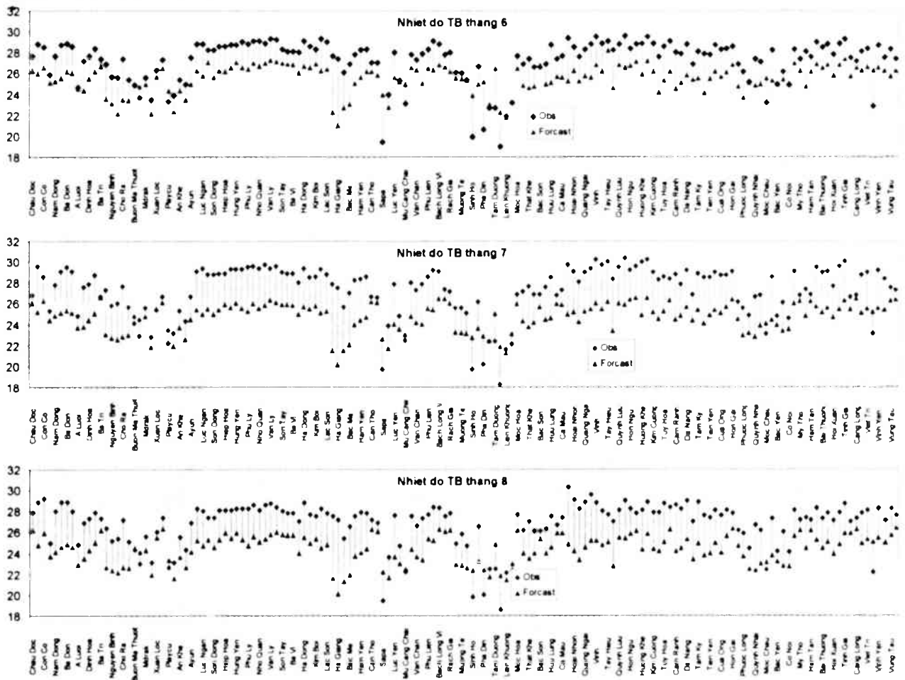
Hình 7. Nhiệt độ trung bình tháng theo số liệu quan trắc (chấm xanh) và mô phỏng của RegCM–CAM (chấm đen).
