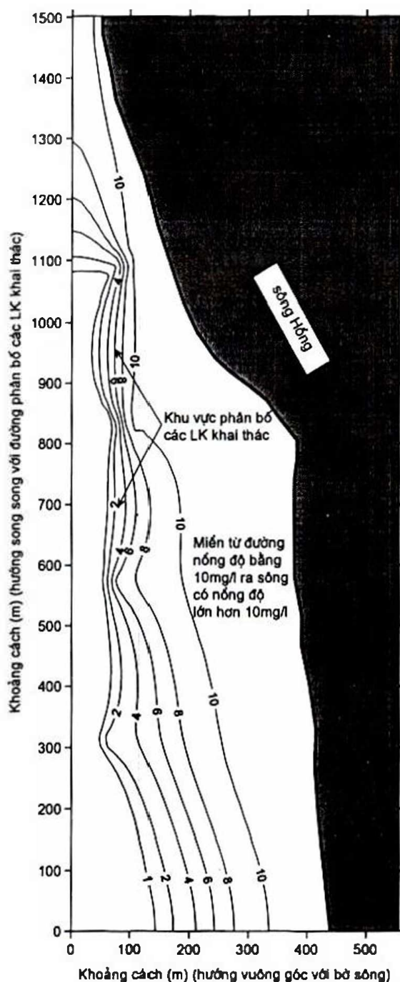
Hình 8. Phân bố nồng độ \text{NO}_3 sau 6 tháng.
